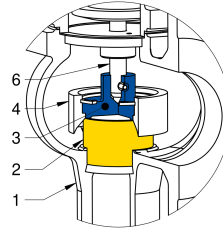
630 Исполнение 51-58
