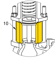
610, 630 Исполнение 01-08
